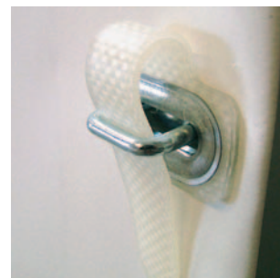
Die Seitenplanen werden mittels Ösenkrampen und Steckstrippen am Gerüst befestigt
