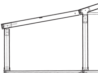
Bewirtungsanbau beidseitig 3,0 m oder 4,0 m tief anbaubar.
