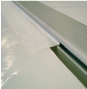
Einfacher wasserdichter Planeneinzug durch Kedernuttechnik
